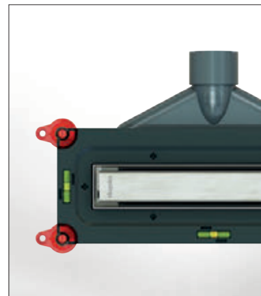
Ενσωματωμένα αλφάδια
